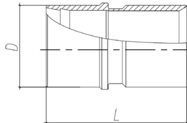
Рисунок 2.10. Монтажная гильза
