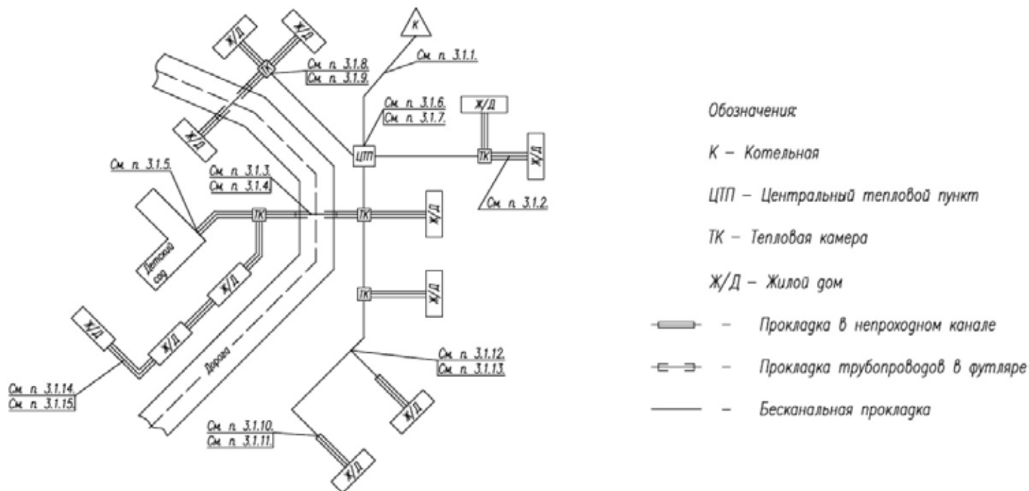
Рисунок 3.1. Пример схемы тепловой сети
