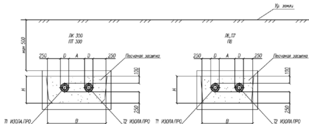
Рисунок 3.3. Прокладка труб в непроходных каналах
