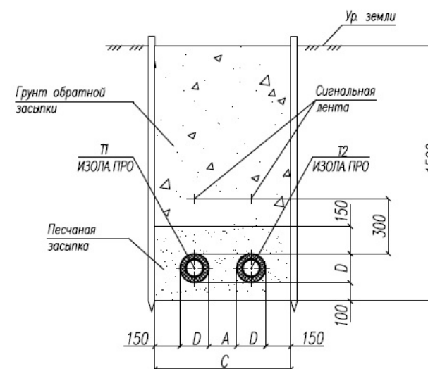
Рисунок 3.2. Прокладка труб в траншее
