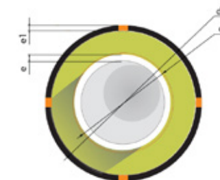
Рисунок 2.4. Размеры труб ИЗОЛА-Т95
