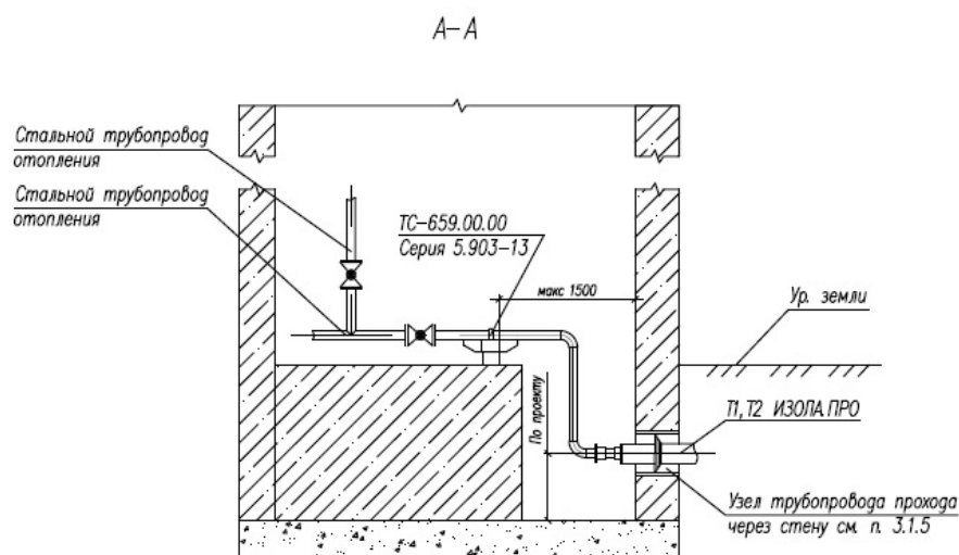
Рисунок 3.10. Узел ввода труб в ЦТП (2-х трубная прокладка)
