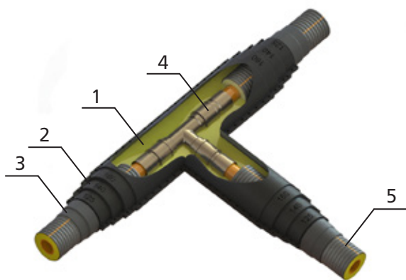
Рисунок 2.13.1. Комплект для изоляции тройника
