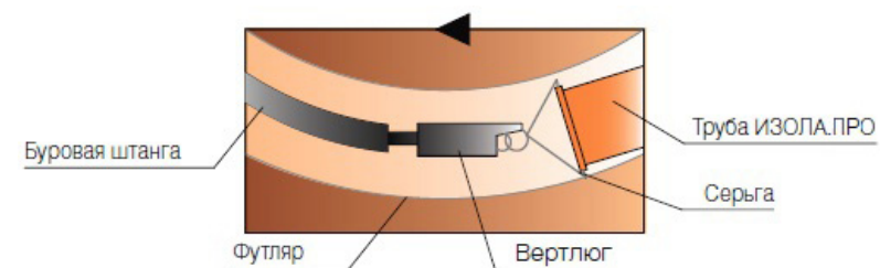
Рисунок 3.8. 4 этап горизонтального направленного бурения
