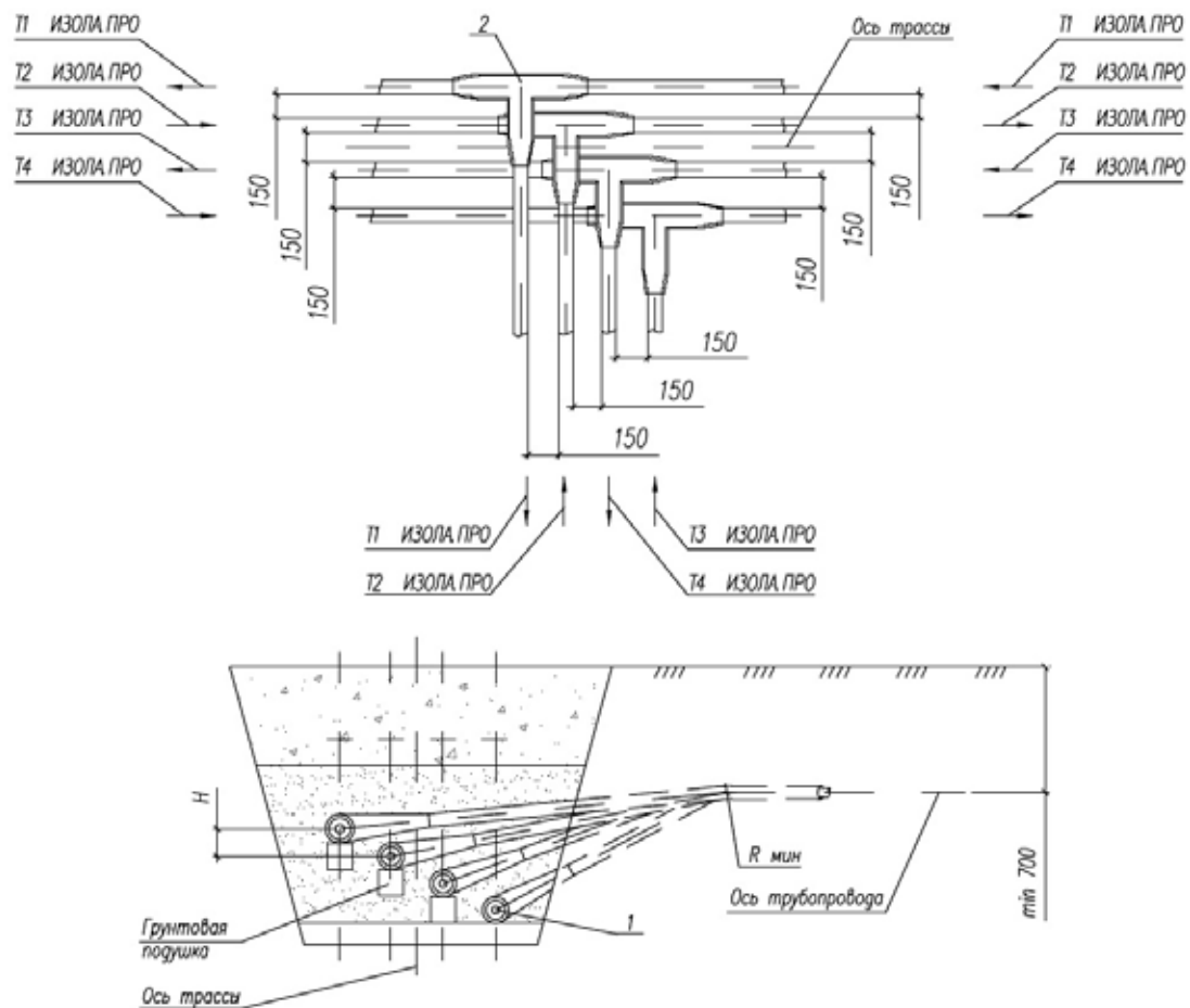
Рисунок 3.19. Тройниковое бесканальное ответвление труб (4-х трубная прокладка)
