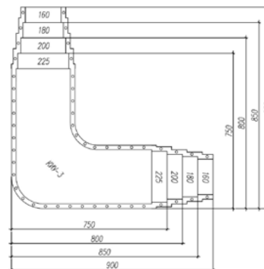
Рисунок 2.14.3. Размеры кожуха комплекта КИУ-3
